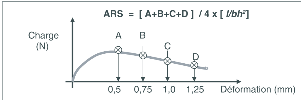
Figure 3 Charge - Courbe de déflexion (ASTM C 1399)
