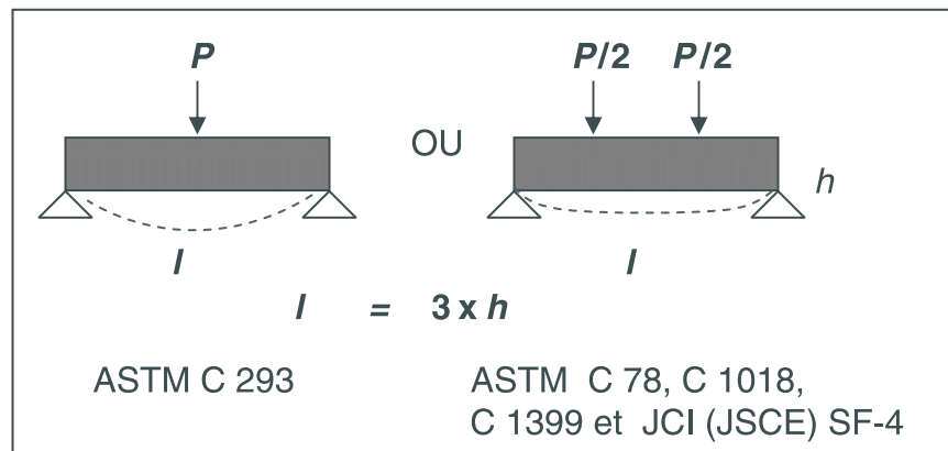
Figure 4 Essais normalisés de résistance à la flexion
