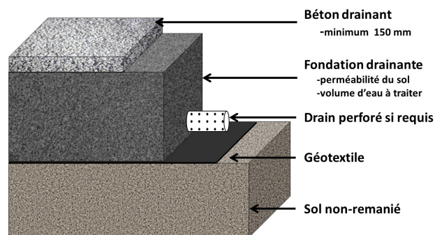
FIGURE 2 Coupe type d'un béton drainant
