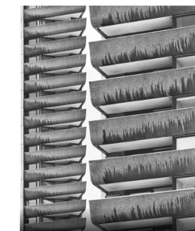
FIGURE 10 Gestion du ruissellement de l'eau
