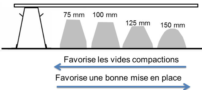
FIGURE 11 Influence de la fluidité sur les risques d'occurrence de vides de compaction
