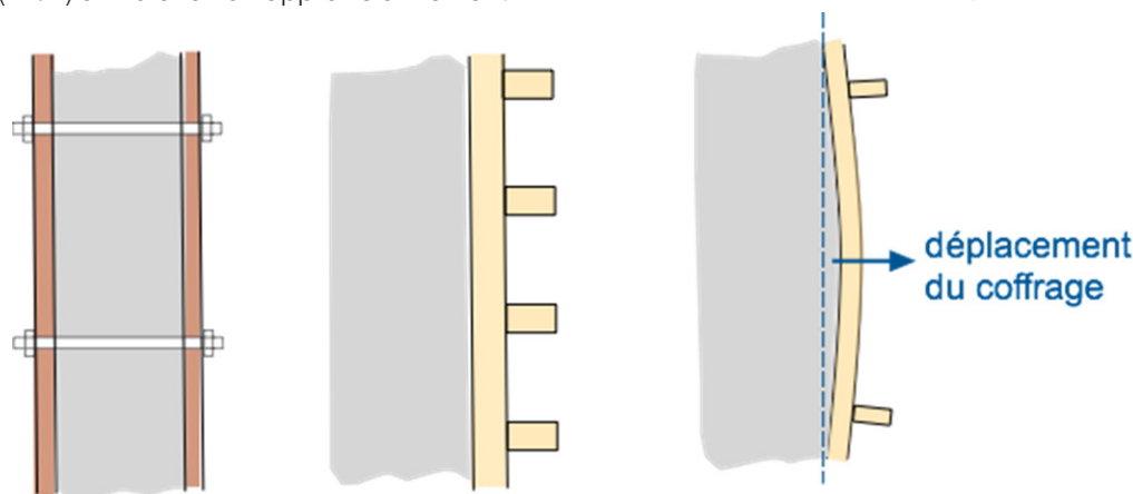
FIGURE 14 Rigidité et contreventement des coffrages (8)
