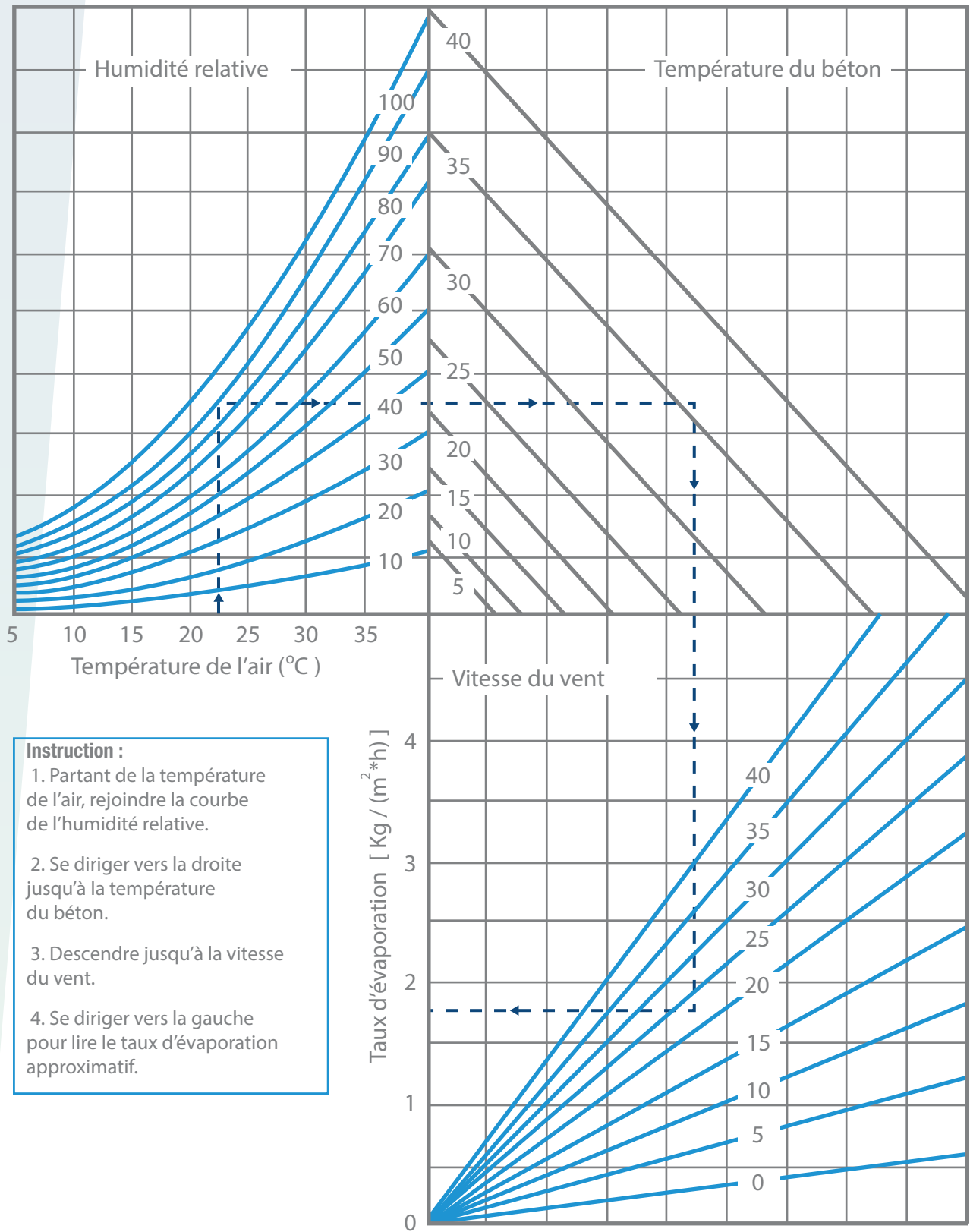
FIGURE 3 Évaluation du taux d'évaporation de l'humidité d'une surface de béton recouverte d'eau 7
