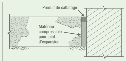
FIGURE 3 Joint de désolidarisation
