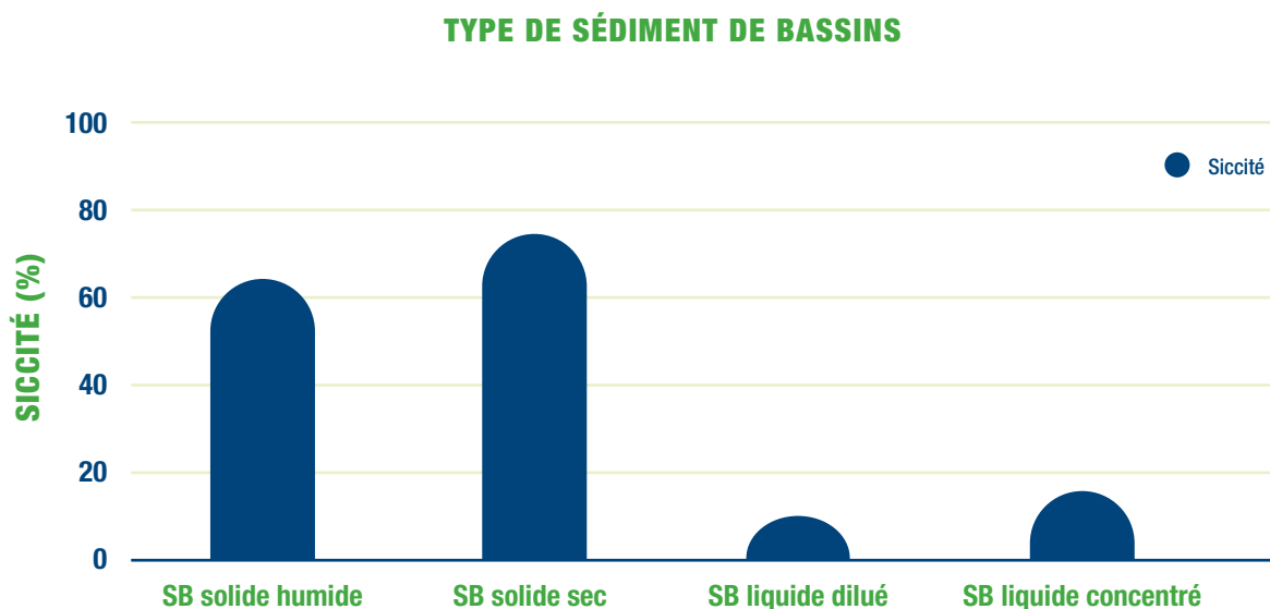
FIGURE 2 — Siccités moyennes (teneurs en solides) minimales et maximales ciblées pour la valorisation agricole des sédiments de bassins
